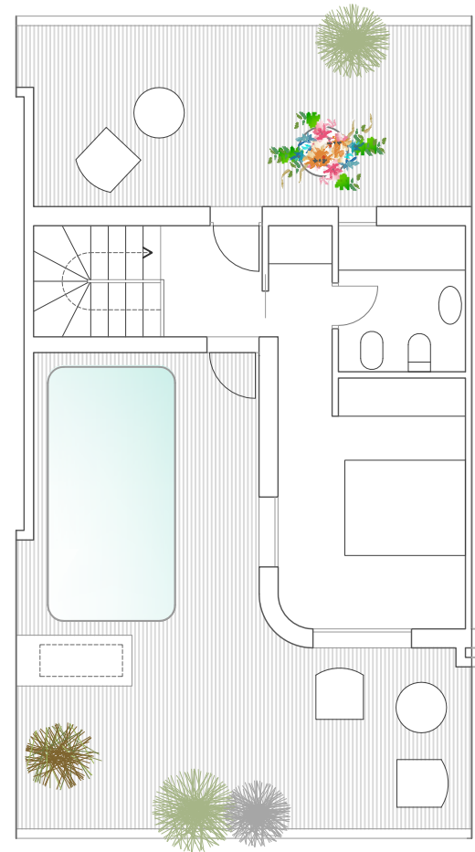
PLANTA ALTA DÚPLEX
